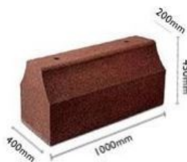
Rys. 1. Wymiary urządzenia
