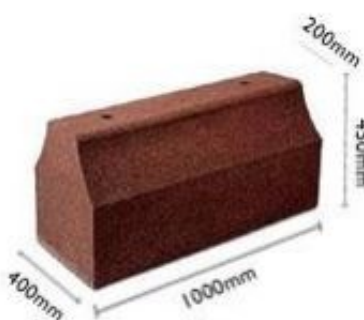
Rys. 1. Wymiary urządzenia
