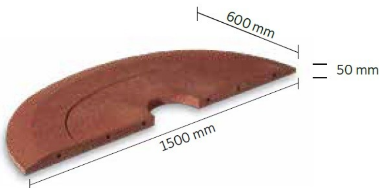
Rys. 1. Wymiary kołnierza
