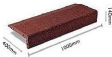
Rys. 1. Wymiary osłony
