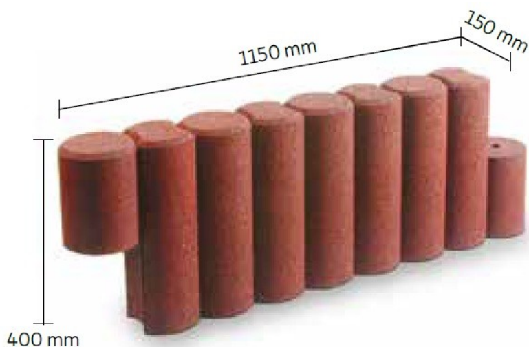
Rys. 1. Wymiary palisady
